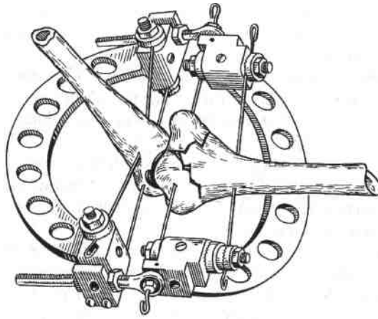
Рис. 11.7. Применение аппарата Волкова — Оганесяна при чрезмышечковом переломе плечевой кости.
