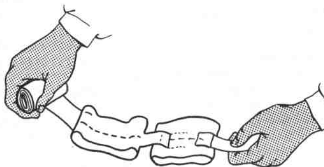
Рис. 6.7. Индивидуальный перевязочный пакет.
