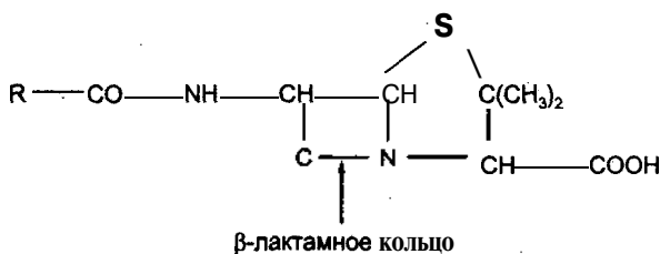
Рис. 32. Молекула пенициллина.
