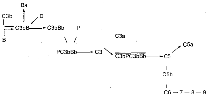
Альтернативный путь активации комплемента
