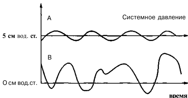
Рис. 25.6. Кривые изменения давления при назальном СРАР, проводимом с помощью разных систем.
